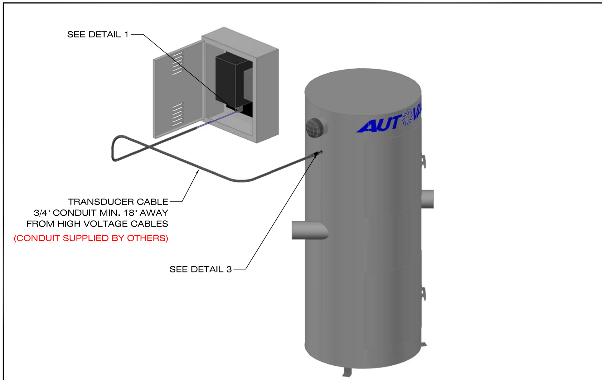
5 ELEVATION VIEW - N.T.S.
